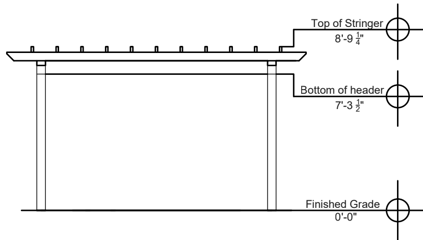
End Elevation
