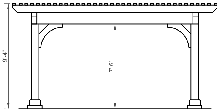
End Elevation
