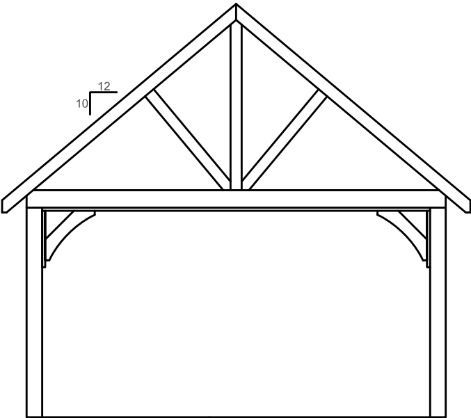
End Elevation
