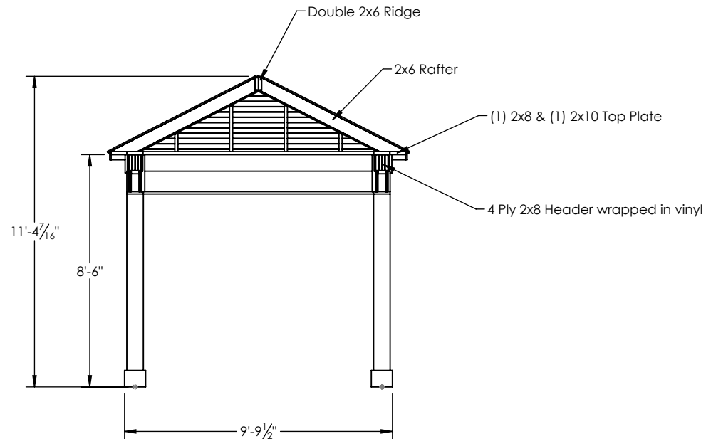
SECTION A-A
